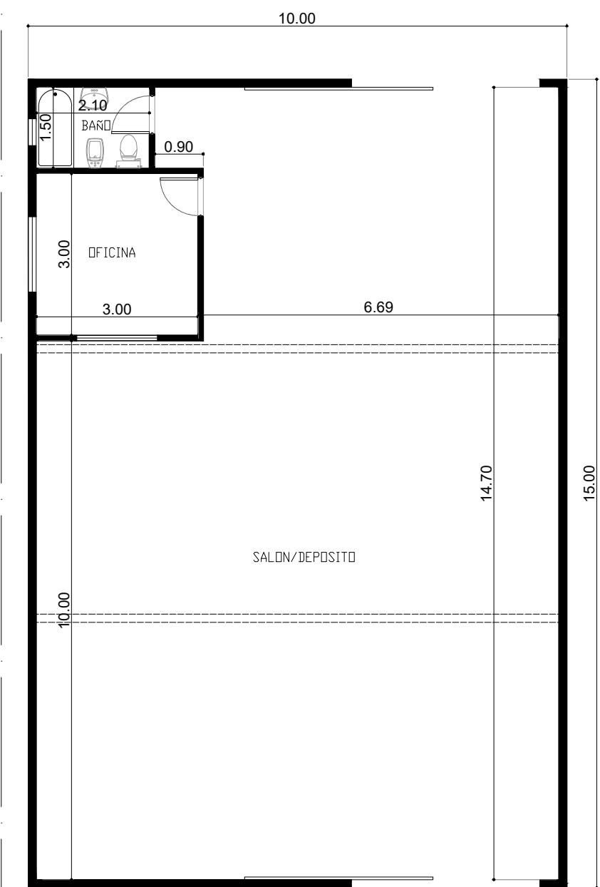
PLANTA GALPON
